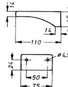
Wandhalter BS 788
