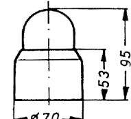
Aufputzleuchte 022
