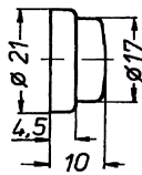
Nr. 8-SL 3 Schraublinse
