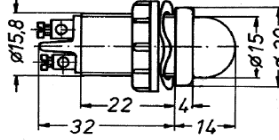
Nr. 8-D2 Schraublinse
