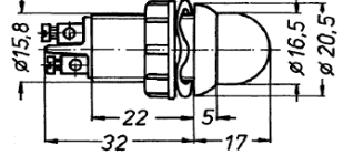
Nr. 8-D1 Schraub / Schnapplinse
